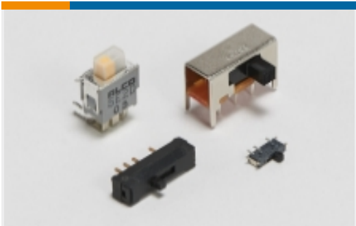
滑动开关(63)
