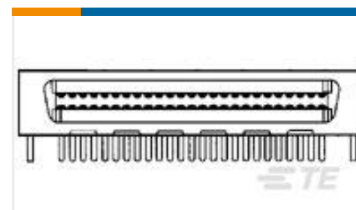
TE 产品编号 1734037-2 Champ 050 series, 80pos, Au over PdNi
