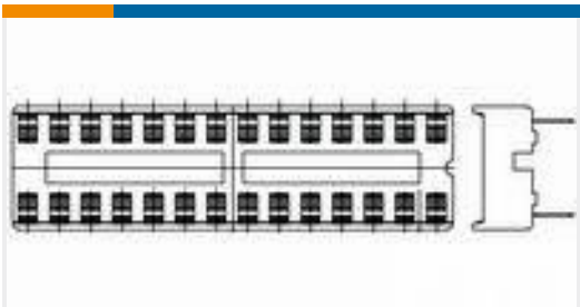
TE 产品编号1-2199298-2 8P,DIP SKT,300 CL,LDR,PB FREE
