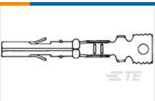
TE 产品编号794001-2 MR RECPT AU PHBZ LP 26-24
