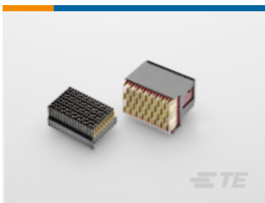
TE 产品编号 2332816-1 RA Plug Assy Left End Multigig RT 3
