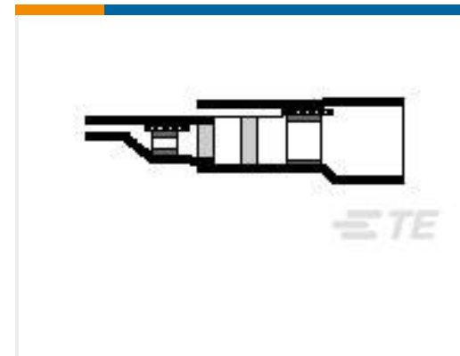
TE 产品编号 443631-000 B-040-30-N
