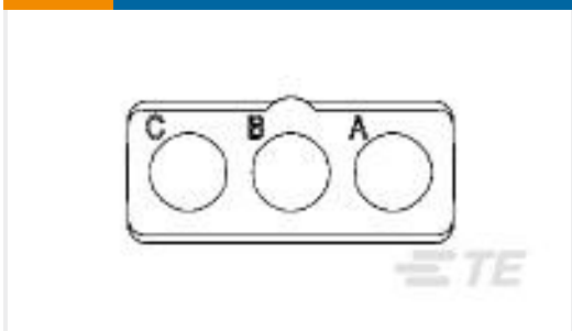
TE 产品编号1738095-1 Asy,Insert,Socket, GPRBNC3SB
