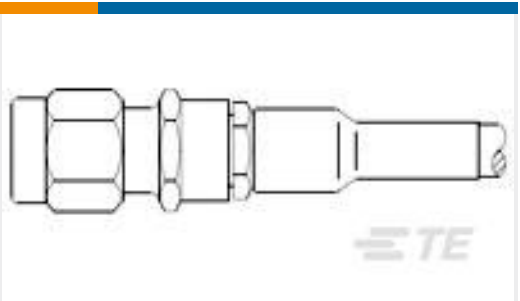
TE 产品编号1051780-1 SMA CABLE PLUG 2031 8025 92
