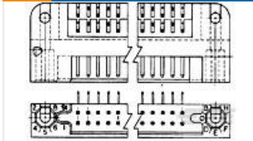
TE 产品编号1-531720-3 2 ROW BOX PIN 150 POS R/A
