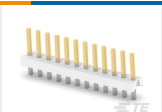
TE 产品编号 4-644756-2 12P MTA156 HDR ASSY STR AU LF
