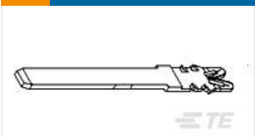
TE 产品编号1601112-2 131-187-014=TAB,110X032,STD SMZ
