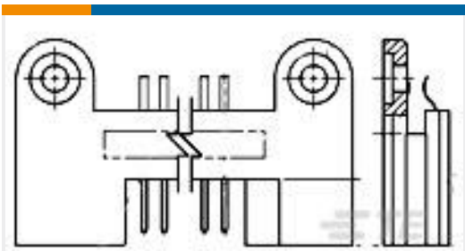
TE 产品编号1-530785-5 BOX PIN HDR ASSY 20 PS 075 CL
