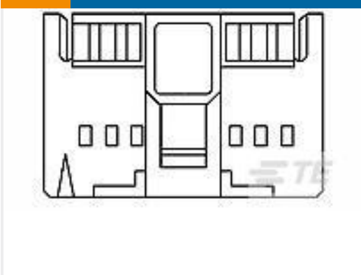
TE 产品编号103681-4 14 MTE COUPLING SHRD DR
