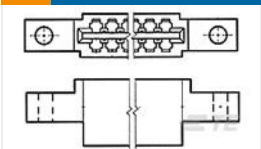
TE 产品编号E74153-000 T1K-508064-10-9
