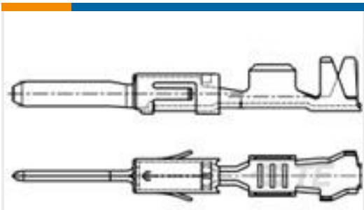
TE 产品编号963900-2 TAB A 1.6x0.6 CONTACT CF SRC Sn
