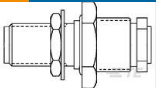
TE 产品编号1051026-1 SMA BULKHEAD JACK 2004 8005 90
