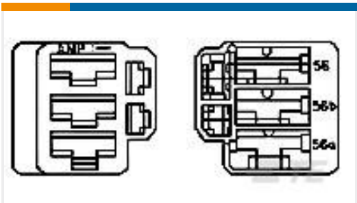
TE 产品编号880191-1 5W FASTIN-ON REC. H
