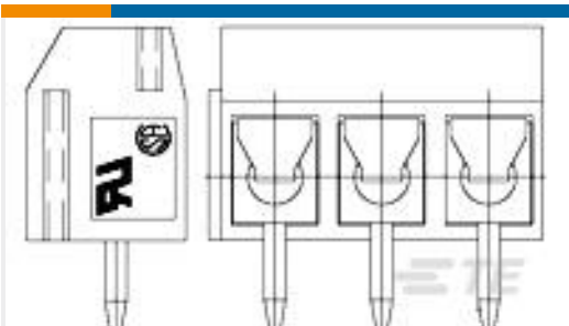
TE 产品编号1776266-2 Vert Side Wire Entry, 5.0mm, G
