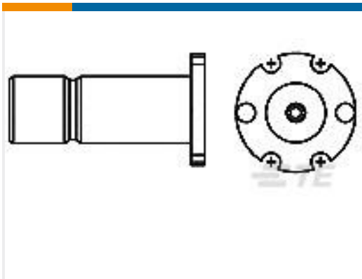
TE 产品编号1080440-1 SCD,5166 5006 09,SMB
