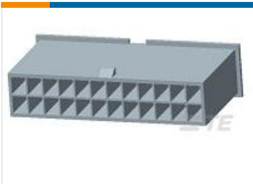
TE 产品编号1-1969598-6 16P FH PLUG VAL-U-LOK V2
