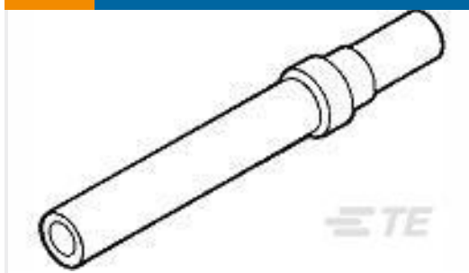
TE 产品编号1218267-3 CONT,CRIMP SKT,20-24AWG,SZ 20
