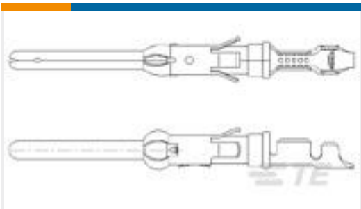
TE 产品编号163085-9 .062 DIA PIN ASS 3+
