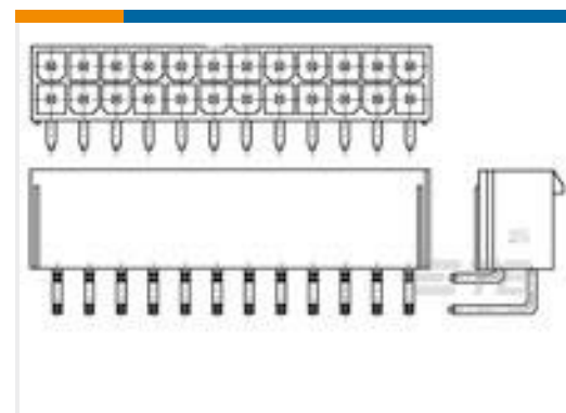
TE 产品编号1586041-6 6P VAL-U-LOK R/A HDR V2
