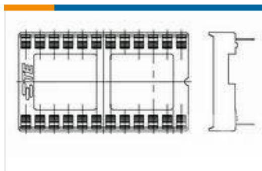
TE 产品编号 1-2199299-5 40P, DIP SKT, 600 CL, LDR, PB FREE
