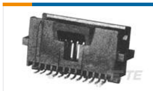
TE 产品编号104549-1 10 SYS50 SURFMNT HDR DRST SHRD
