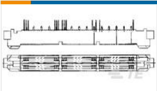
TE 产品编号 5767055-2 MICT,R/APLUG,ASSY,76,PDNI
