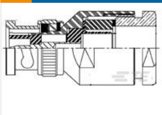
TE 产品编号1-1478405-0 BNC Str Plg PS 75Ohm Silver URM202 /U, 18
