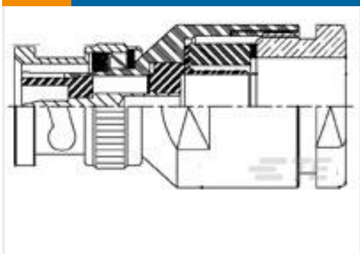
TE 产品编号1-1478402-0 BNC Str Plg PS 50Ohm Silver RG174A /U, 18
