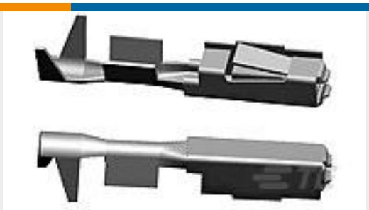
TE 产品编号968678-2 MPQ2,8 Sn rec LL unseal. 0,35-0,5
