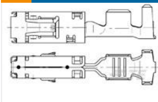
TE 产品编号967542-1 SENSOR FLA-KONT 2,8
