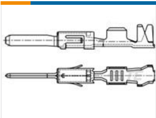
TE 产品编号963900-1 TAB A 1.6x0.6 CONTACT CS SRC Sn
