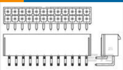
TE 产品编号1-1586041-4 14P VAL-U-LOK R/A HDR V2
