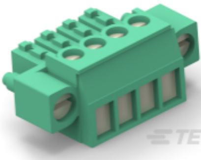
TE 产品编号 284511-6 6 POS TERMI-BLOK PLUG C. VITI
