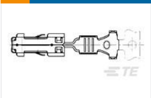
TE 产品编号1703034-2 SENSOR CONTACT 2,8
