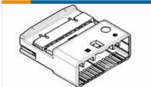
TE 产品编号1379681-1 24W TAB HSG ASSY BLACK
