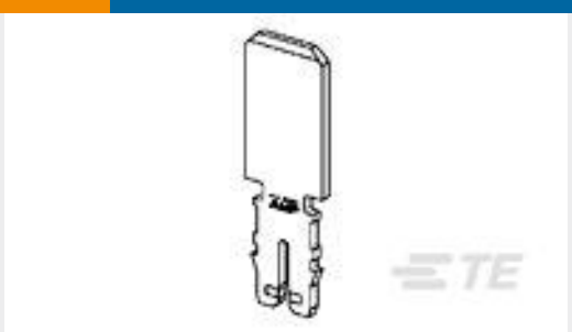
TE 产品编号136826-1 SPEC TAB MAG MATE 6.35
