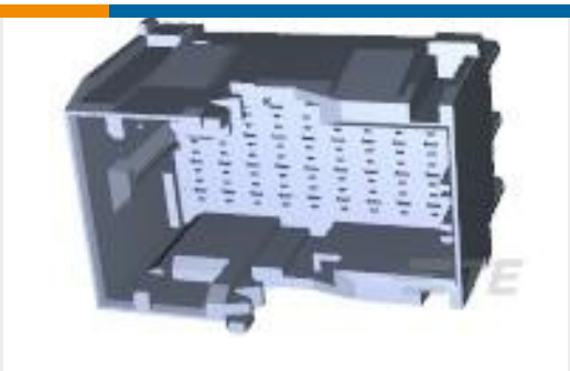
TE 产品编号1-1718492-1 1.5MM TAB HSG 36 POS ASSY
