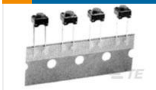
TE 产品编号147997-1 FSM4JART=SWITCH,TACTILE, 6MMX6M
