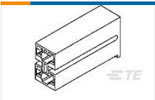
TE 产品编号1-172210-4 3P PL MK-2 187(4.8 MM) HOUSING REC
