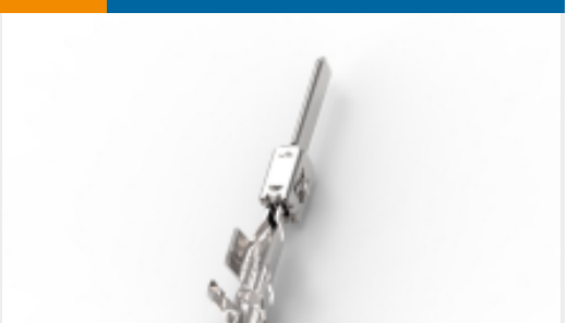
TE 产品编号2-2141600-2 TAB 2.8x0.8 CONTACT CF SRC Ag
