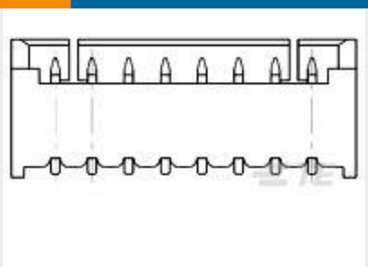
TE 产品编号1-1734829-1 1.25 WTB HDR DIP, 11 POS
