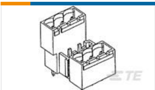
TE 产品编号1-284065-6 TERMI-BLOK HDR 180, 5,08MM P.M
