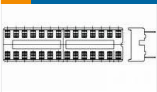
TE 产品编号1-2199298-3 14P,DIP SKT,300 CL,LDR,PB FREE
