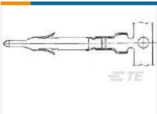
TE 产品编号170363-3 MINI UNIVERSAL M-N-L PIN LP
