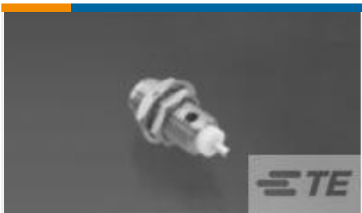
TE 产品编号1051032-1 SMA BULKHEAD JACK 2004 8207 92
