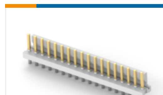
TE 产品编号 4-644766-8 18P MTA156 HDR ASSY STR SQ LF
