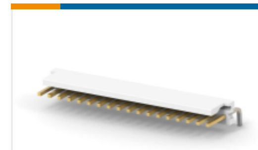
TE 产品编号 4-641121-8 18P MTA156 HDR ASSY FL/RA LF
