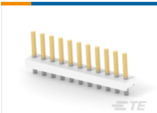
TE 产品编号 4-641203-1 11P MTA156 HDR ASSY PL 30AU LF
