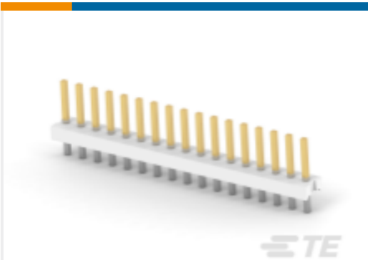
TE 产品编号 4-644756-7 17P MTA156 HDR ASSY STR AU LF
