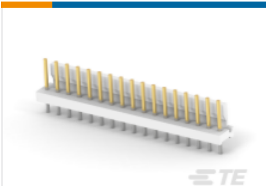
TE 产品编号 4-644760-7 17P MTA156 HDR ASSY FL ST LF
