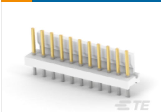
TE 产品编号 4-644760-1 11P MTA156 HDR ASSY FL ST LF
