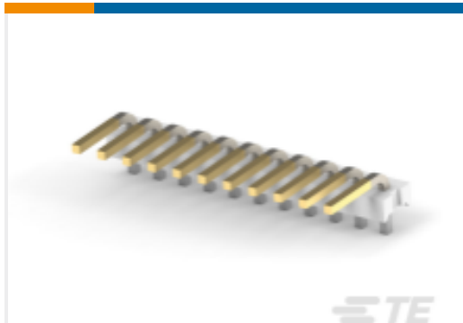
TE 产品编号 4-641204-1 11P MTA156 HDR ASSY PL 30AU LF
