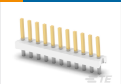
TE 产品编号 4-644756-1 11P MTA156 HDR ASSY STR AU LF
