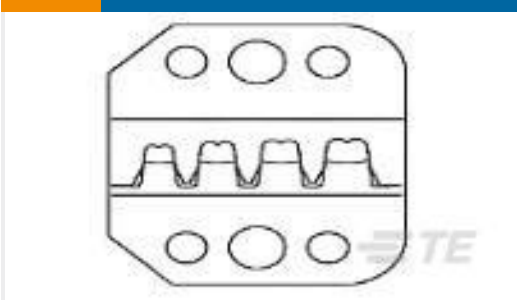
TE 产品编号58641-2 PROCRIMP DIE MOD IV
