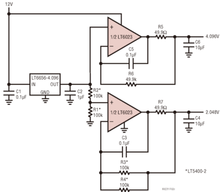
微功耗参考分频器/缓冲器
