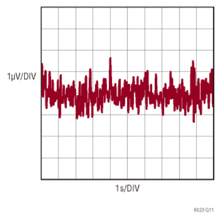
0.1Hz 至 10Hz 电压噪声
