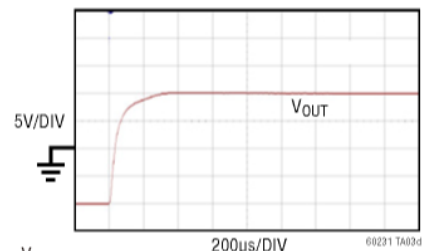
20V 输出阶跃响应
