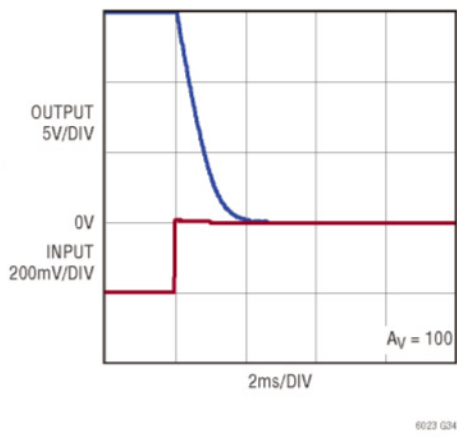
负输出过驱恢复
