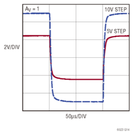
大信号瞬态响应 (5V 阶跃)
