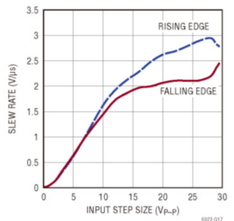
压摆率与输入阶跃的关系
