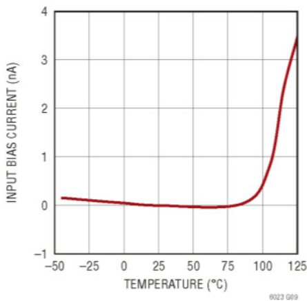
输入偏置电流与温度的关系
