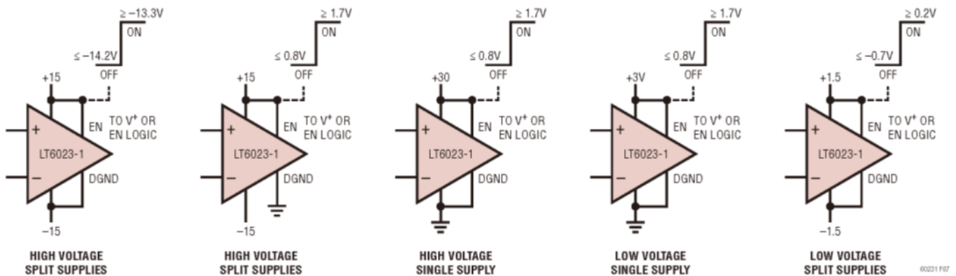
图 7. LT6023-1 使能引脚控制示例
