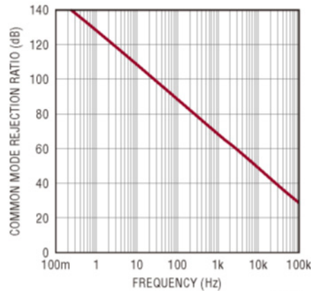
CMRR 与频率的关系
