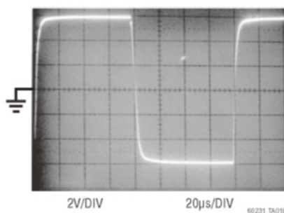
多路复用缓冲器响应，12V 阶跃
