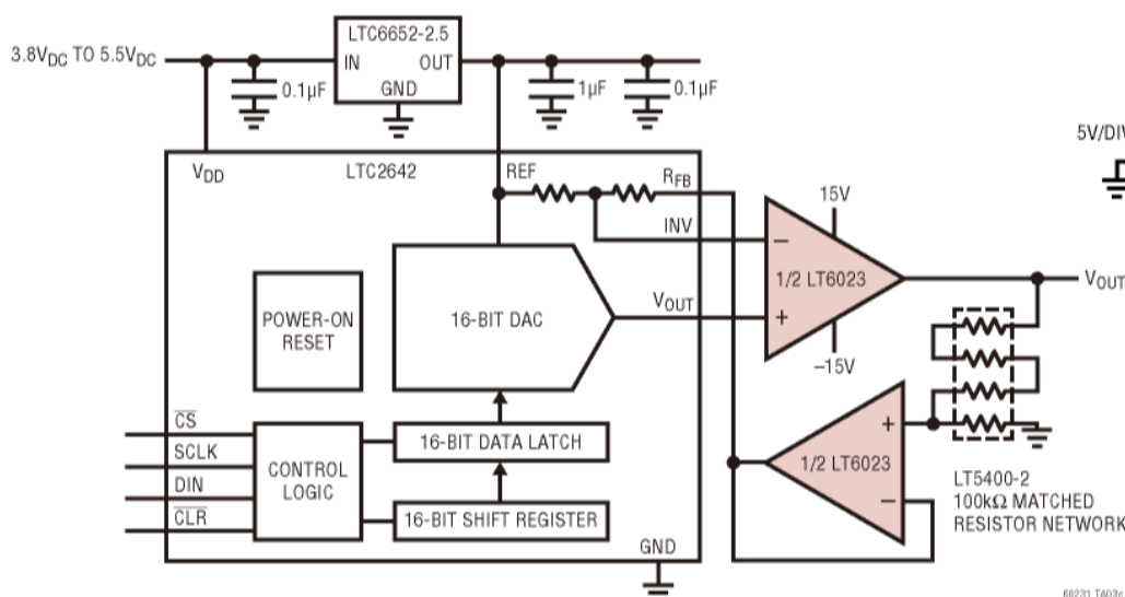
提供 \pm 10V 输出摆幅的 16 位 DAC
