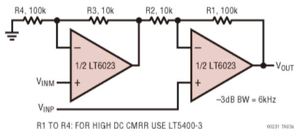
11 倍增益仪表放大器
