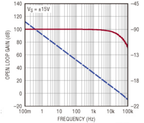
开环增益和相位与频率的关系
