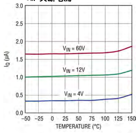
V_{IN} 关断电流
