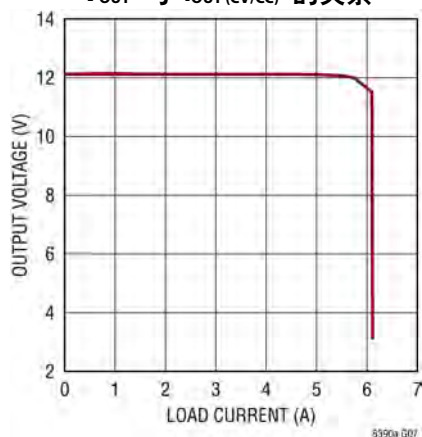
V_{OUT} 与 I_{OUT} (CV/CC) 的关系
