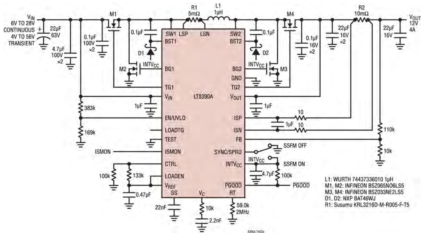
95% 效率、48W (12V 4A)、2MHz 降压-升压稳压器
