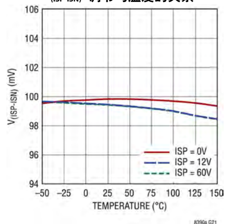
V_{(ISP-ISN)} 调节与温度的关系
