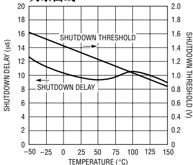
关断延迟和门限与温度的关系曲线
