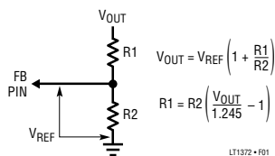
图 1：正输出电阻分压器
