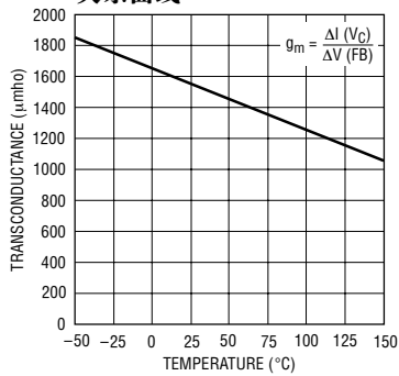
误差放大器跨导与温度的关系曲线
