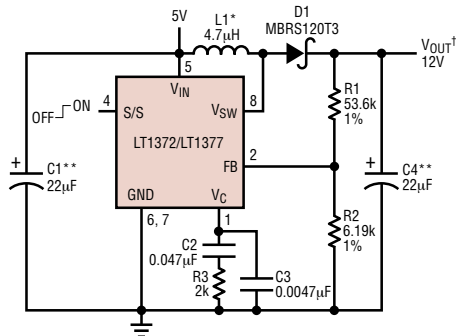
5V 至 12V 升压转换器
