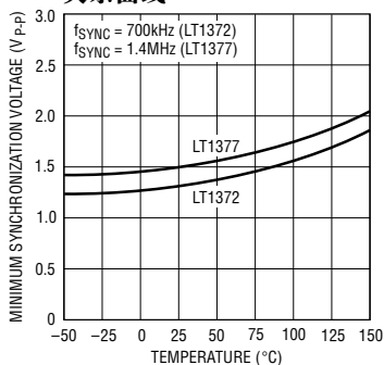
最小同步电压与温度的关系曲线
