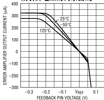
误差放大器输出电流与反馈引脚电压的关系曲线
