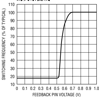
开关频率与反馈引脚电压的关系曲线
