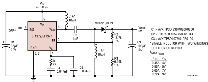
双锂离子电池至 5V 的 SEPIC 转换器
