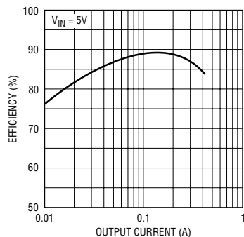
12V 输出效率
