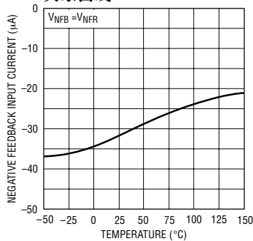
负反馈输入电流与温度的关系曲线
